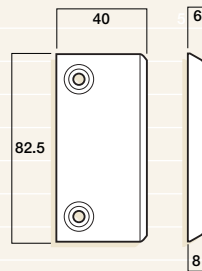
No lug body W8215
